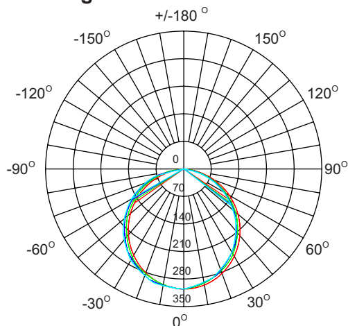
Diagrama fotometrica
