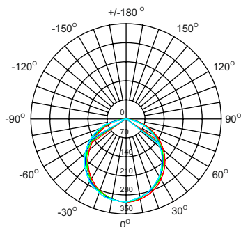
Diagrama fotometrica
