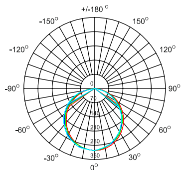
Diagrama fotometrica
